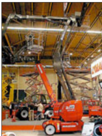
Die neue Manitou 150 AETJ
